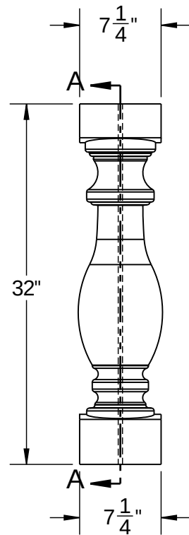
ELEVATION
