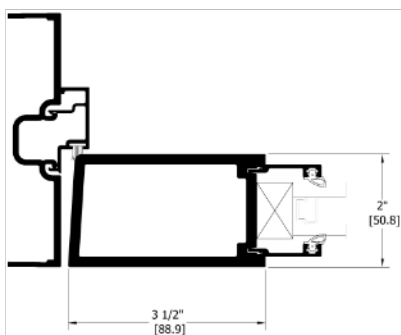
MEDIUM STILE
