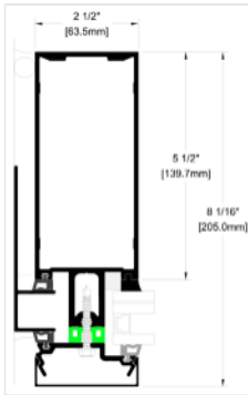
Thermal Separator
