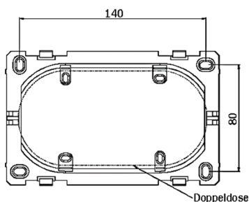
Abbildung Montagerahmen an bauseitiger Doppeldose
