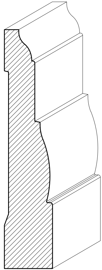
SWCA38 \frac{7}{8}" \times 4\frac{5}{16}"
