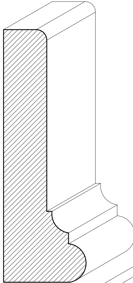
SWCA02 1\frac{3}{8}" \times 4\frac{1}{2}"
