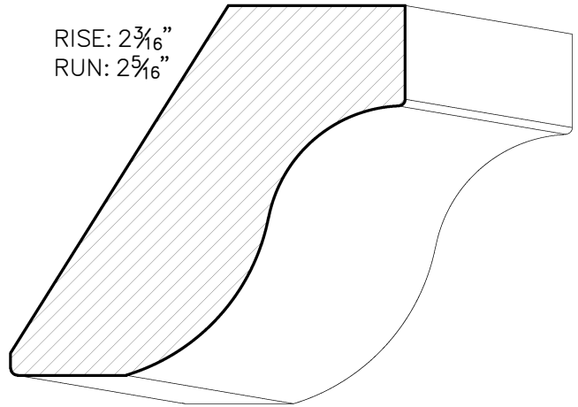
SWCR34 1\frac{1}{8}" \times 3"
