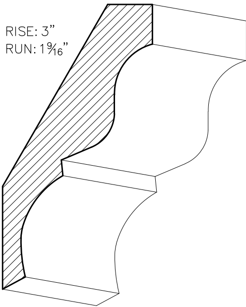
SWCR27 \frac{3}{4}'' \times 3\frac{3}{8}''
