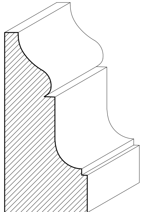
SWCA30 1\frac{3}{8}" \times 3"
