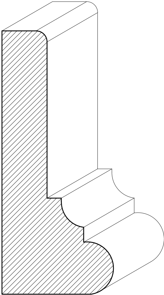
SWCA01 1\frac{7}{8}" \times 4\frac{1}{2}"
