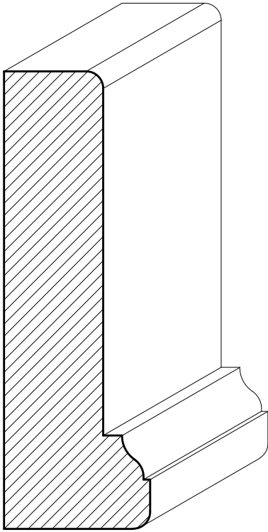
SWCA11 1\frac{1}{8}" \times 3\frac{1}{2}"
