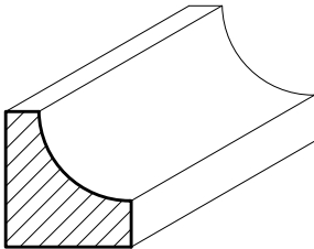
SWQR13 \frac{5}{8}" \times \frac{5}{8}"
