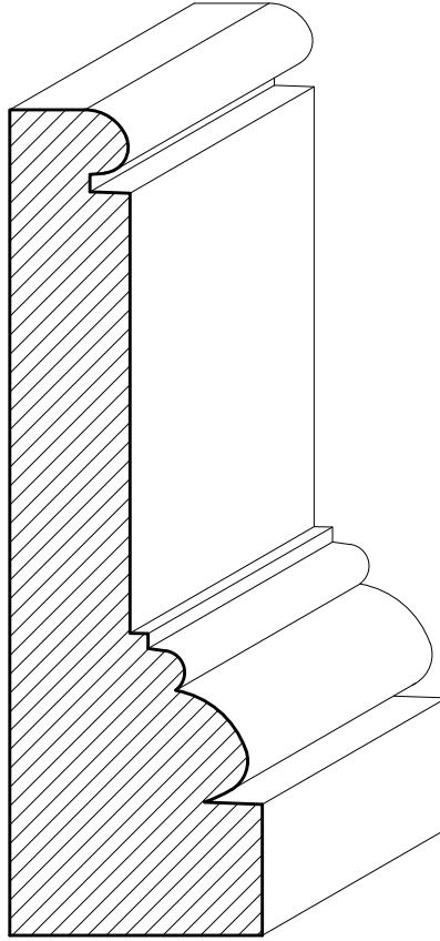
SWCA37 1\frac{3}{16}" \times 3\frac{7}{8}"
