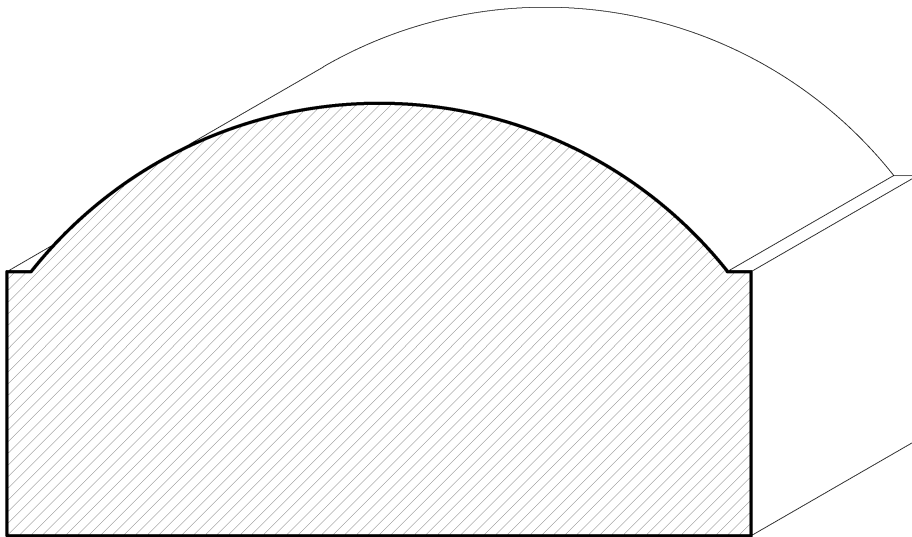
SWHR12 3\frac{7}{8}" \times 2\frac{1}{2}"
