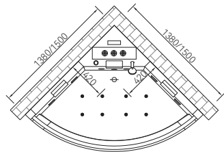
Q322N 1380*1380*630mm 1500*1500*600mm
