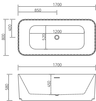
Q191 1700*800*580mm
