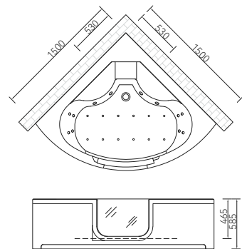
Q374 1500*1500*585mm
