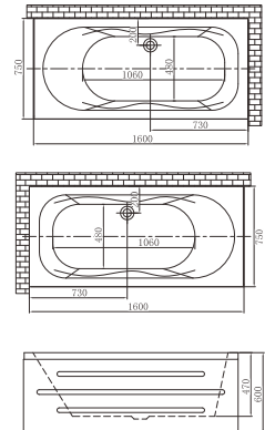
Q109 (L/R) 1600*750*600mm
