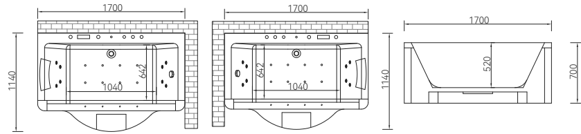
Q420 (L/R) 1700*1140*700mm
