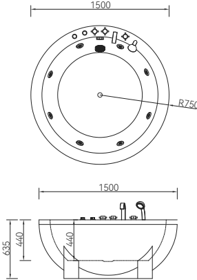
Q414 1500*1500*635mm
