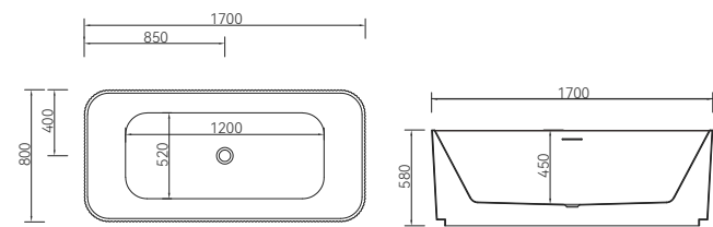
Q187 1700*800*580mm
