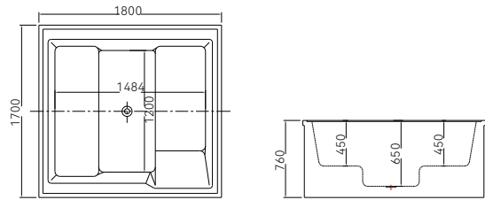
Q457 1800*1700*760mm
