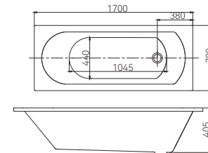
Q426A-170 1700*700*420mm
