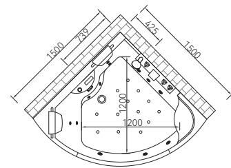
Q437 1500*1500*650mm
