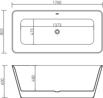
Q183 1700*800*600mm
