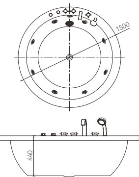
Q414A 1500*1500*440mm
