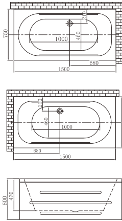
Q108 (L/R) 1500*750*600mm
