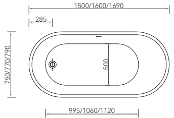
Q163A-17 0 1690*790*600mm
