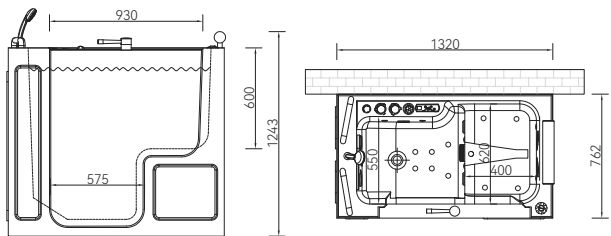
Q358 (L) 1320*762*1143mm
