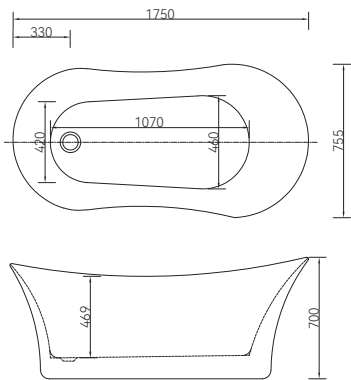
Q167 1750*755*700mm
