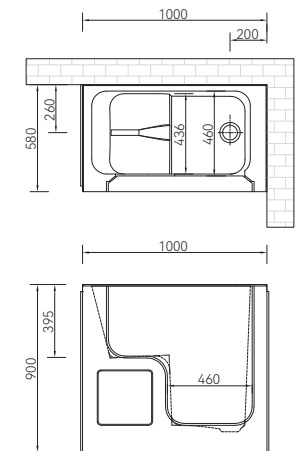
Q372-100 (R) 1000*580*900mm
