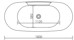
Q336 1800*800*740mm
