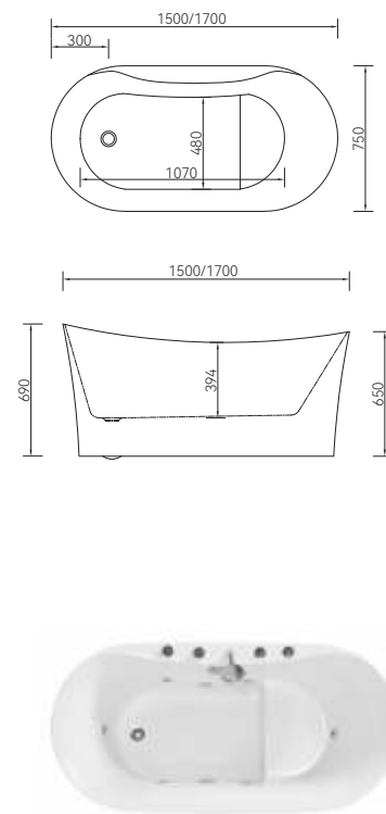
Q193 1500*750*690mm , 1700*750*690mm
