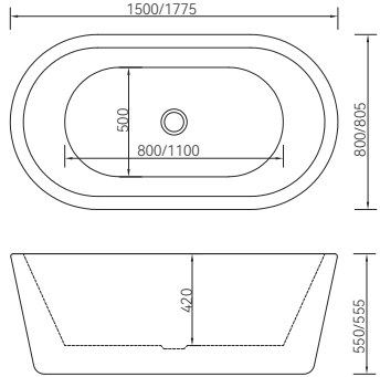
Q166-175 1755*805*555mm
