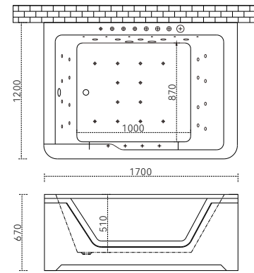
Q450W(L/R) 1700*1200*670mm
