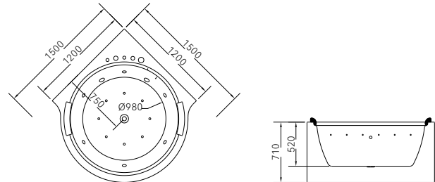
Q452 1500*1500*710mm
