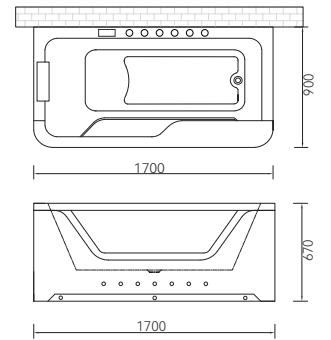
Q449(L/R) 1700*900*670mm
