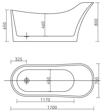
Q197 1700*700*800mm
