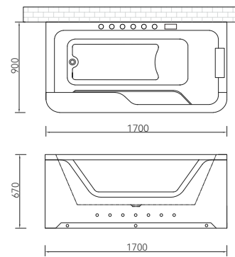
Q449W(L/R) 1700*900*670mm
