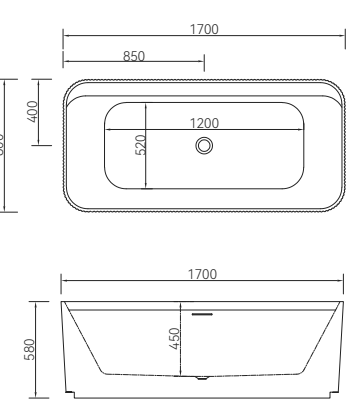
Q187F 1700*800*580mm
