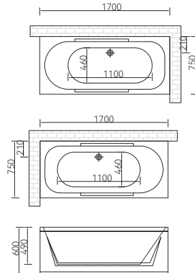
Q111 (L/R) 1700*750*600mm
