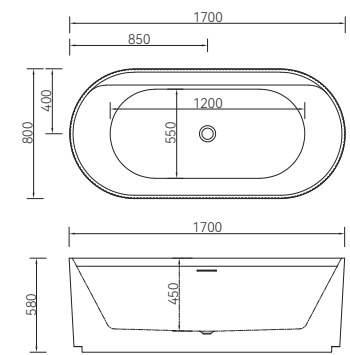
Q186F 1700*800*580mm
