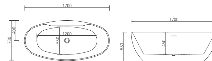
Q185 1700x800x580mm
