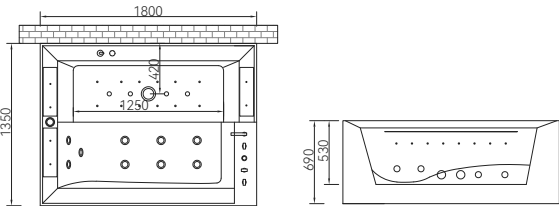
Q439 1800*1350*690mm
