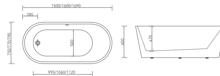
Q163-150 1500*750*600mm Q163-160 1600*770*600mm Q163-170 1690*790*600mm
