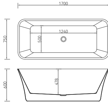
Q182 1700*750*600mm
