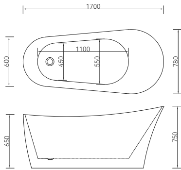
Q156A-170 1700*780*750mm
