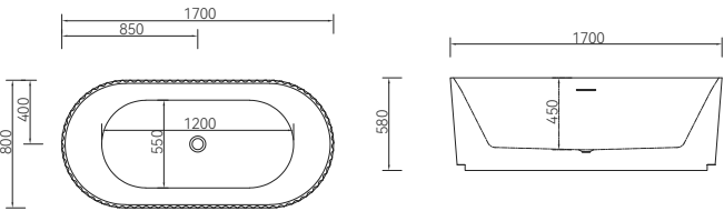
Q190 1700*800*580mm
