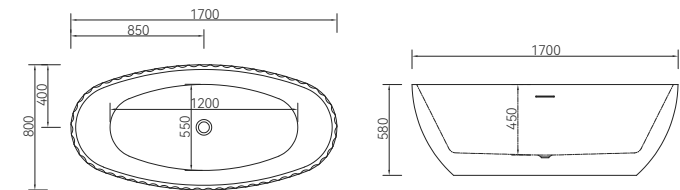
Q326S 1700*800*580mm
