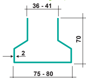
PR 35 - Kg/mt: 3,60
