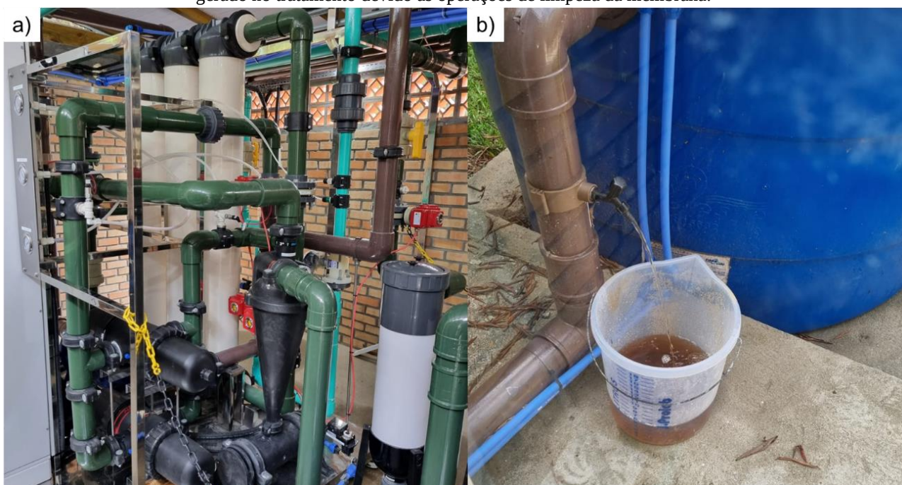
Figura 14 – a) Visão do sistema de membranas de UF instalado na região da Grande Florianópolis. b) Subproduto gerado no tratamento devido às operações de limpeza da membrana.
