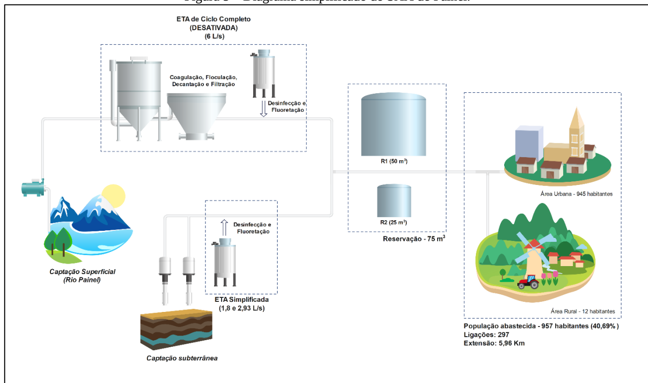
Figura 5 – Diagrama simplificado do SAA de Painel.
