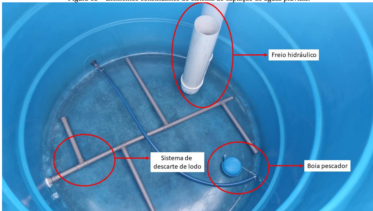
Figura 15 – Elementos constituintes do sistema de captação de águas pluviais.
