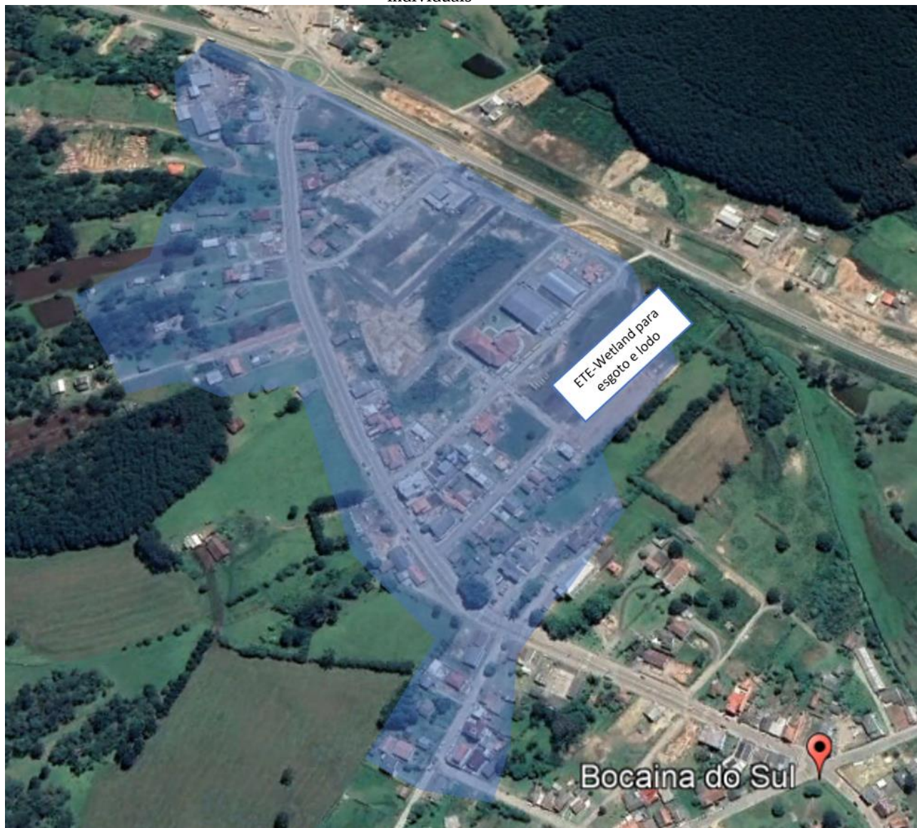
Figura 17 - Bacia de contribuição para o tratamento de esgoto descentralizado e do lodo proveniente dos sistemas individuais
