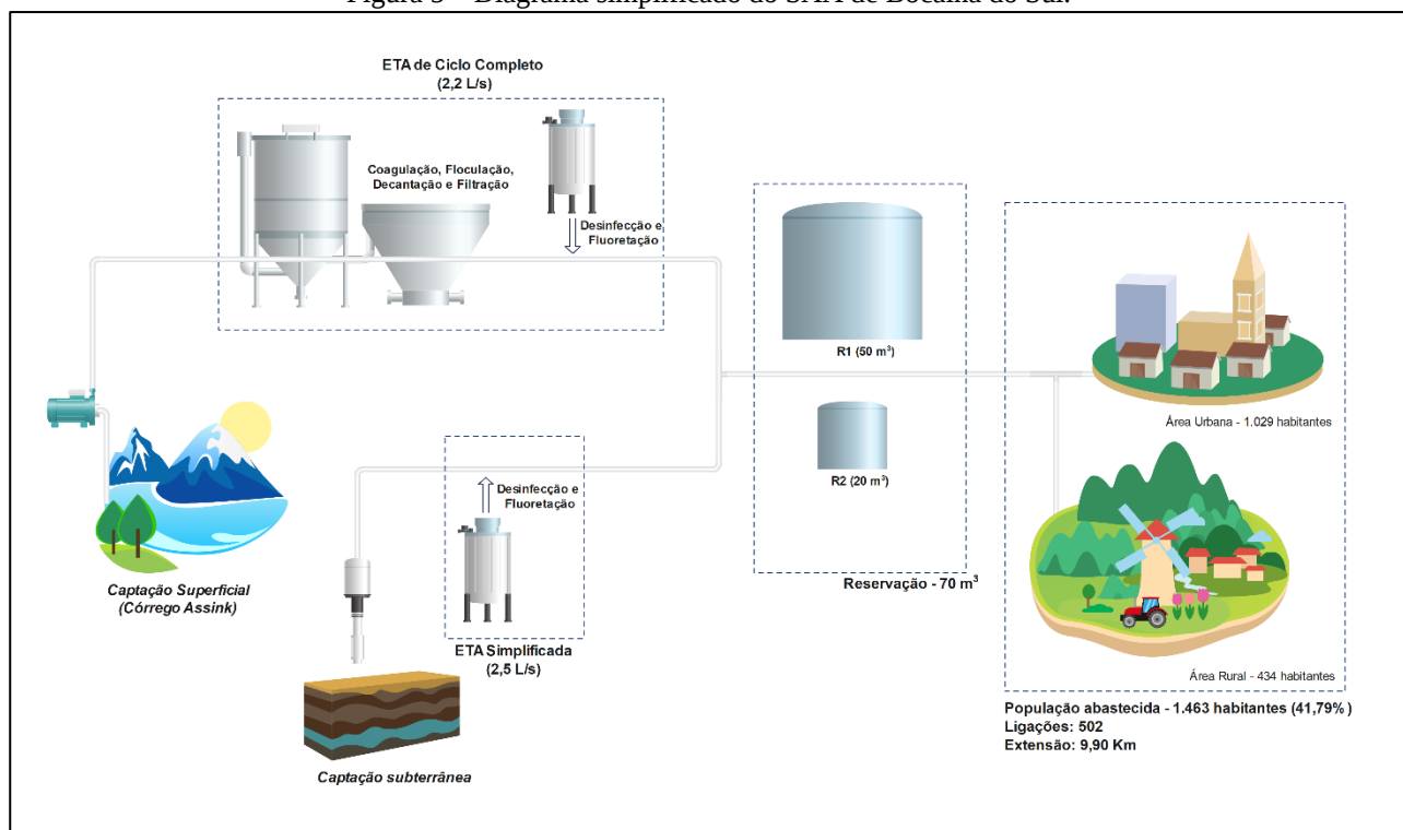
Figura 5 – Diagrama simplificado do SAA de Bocaina do Sul.
