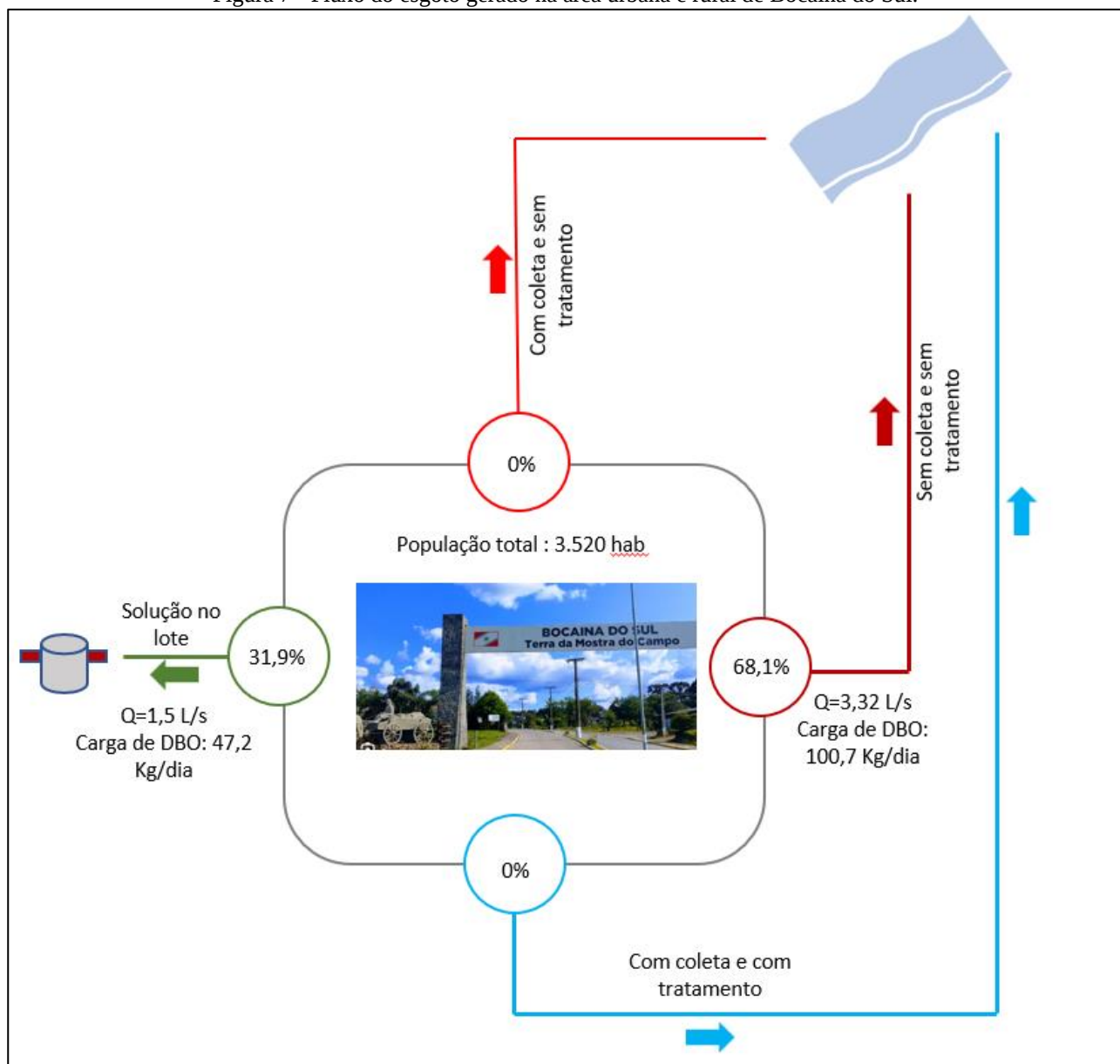
Figura 7 - Fluxo do esgoto gerado na área urbana e rural de Bocaina do Sul.
