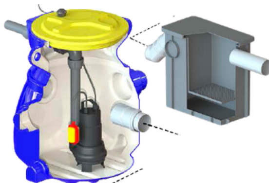
ELEVATÓRIA COMPACTA DE ESGOTO
