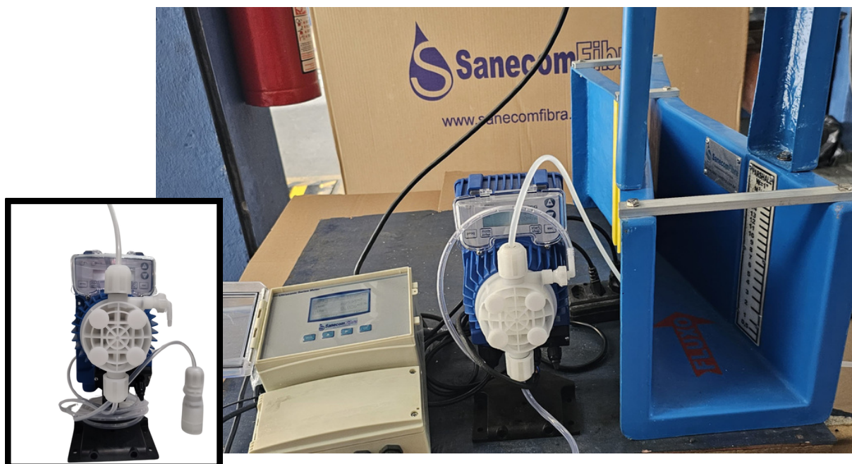
Bomba dosadora com regulagem através do sinal 4-20ma do medidor de vazão
