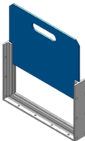
TIPO DE FLANGEAR NO CANAL
