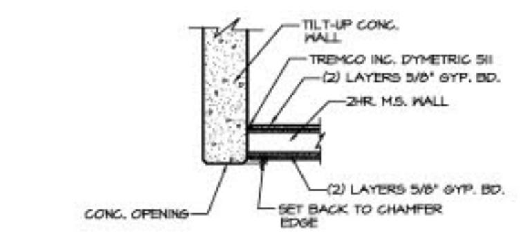
2 2 HR. WALL @ DOORS SCALE: 1/2" = 1'-0"
