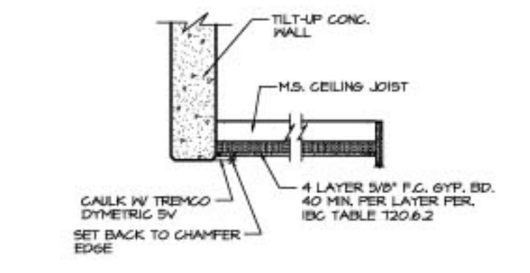
3 2 HR. CEILING @ DOORS SCALE: 1/2" = 1'-0"
