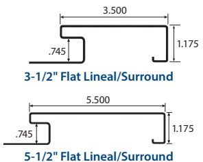
Flat Lineal Surround 20' long 10 pieces per carton 200 linear feet per carton
