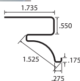
Soffit Cove Moulding 12' 6" long 20 pieces per carton 250 linear feet per carton
