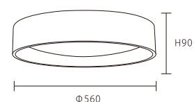
OK 31643 41000 Φ560*H90mm 内含 LED 36W 三段式光色 鋼材 壓克力
