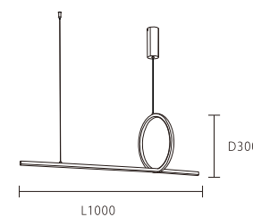
OK 30641 74000 L1000*D300mm 線長: 1500mm 內附 LED 25W 4000K 不銹鋼 壓克力
