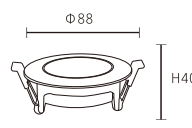
JBR-31075 尺寸 \Phi 88 \times H40 mm 開孔尺寸 \Phi 75 可適用MR16
