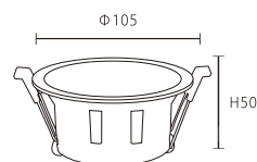
JBR-31092B/W 尺寸 \Phi 105 \times H 50 \text{mm} 開孔尺寸 \Phi 85 可適用MR16
