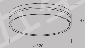
OK 31721/31722 20000 Φ520*H70mm 內含 LED 45W 三段式光色 鋼材 壓克力
