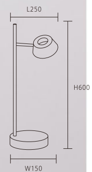
OK 31572 40000 W150*L250*H600mm 線長: 1500mm 內附 LED 8W 3000K 鋼材 附開關
