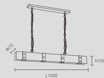
OK 30541 78000 L1000*W75*H100mm 鍊長: 600mm 內附 LED 5W*4 快拆式光源 鋼材 可選3000K/4000K
