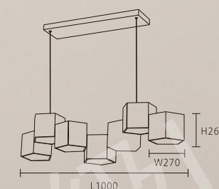
OK 30441 152000 L1000*W270*H260mm 線長: 1500mm 內附 LED 8W*7 4000K 鋼材
