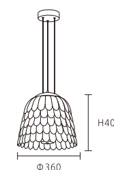
OK 30141 88000 Φ360*H400mm 線長: 1500mm 內附 LED 20W 3000K 鋼材 壓克力
