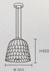
OK 30131 84000 Φ360*H400mm 線長: 1500mm 內附 LED 20W 3000K 鋼材 壓克力
