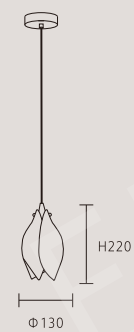
OK 30911 22000 \Phi 130 \times H220\text{mm} 線長: 1500mm E14*1 另計 鋼材 白玻璃
