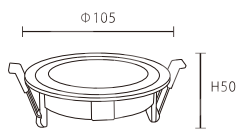
JBR-31076 尺寸 \Phi 105 \times H50 mm 開孔尺寸 \Phi 95 可適用MR16
