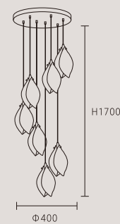
OK 30921 160000 \Phi 400 \times H1700\text{mm} 線長: 1500mm E14*7 另計 鋼材 白玻璃
