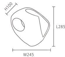
OK 31252 42000 W245*L285*H100mm G4*1 另計 微水泥
