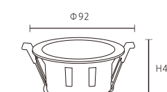
JBR-31082B/W 尺寸 \Phi 92 \times H42 mm 開孔尺寸 \Phi 85
