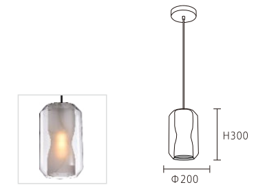
OK 30261 35000 Φ200*H300mm 線長: 1500mm E27*1 另計 玻璃
