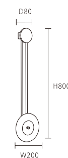
OK 31322 52000 W200*H800*D80mm 内附 LED 6W 3000K 鋼材 水晶砂玻璃
