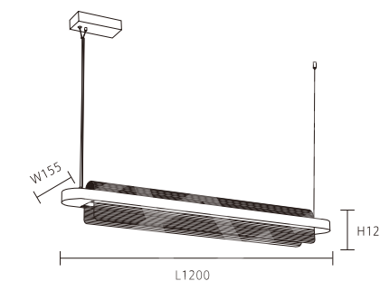
OK 30621 135000 L1200*W155*H125mm 線長: 1500mm 內附 LED 45W 3000K 不銹鋼 壓克力
