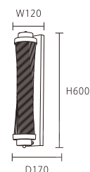
OK 31291/31292 20000 W120*H600*D170mm E14*2 另計 鋼材 水晶玻璃
