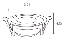
JBR-31093B/W 尺寸 \Phi 95 \times H 35 \text{mm} 開孔尺寸 \Phi 80 可適用MR16
