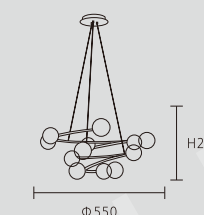
OK 31162 60000 \Phi 550 \times H240 mm 線長:1000mm G9*8 另計 鋼材 玻璃
