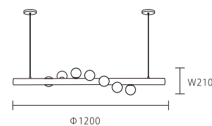
OK 30871 57000 L1200*W210mm 線長: 1500mm G9*7 另計 實木 玻璃
