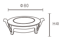
JBR-31077 尺寸 \Phi 80 \times H40 mm 開孔尺寸 \Phi 75 可適用MR16
