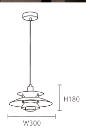
OK 30292 28000 W300*H180mm 線長: 1500mm E27*1 另計 鋼材
