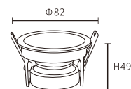
JBR-31074 尺寸 \Phi 82 \times H49 mm 開孔尺寸 \Phi 75 可適用MR16
