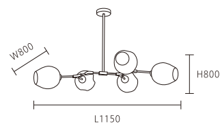
OK 31091 60000 L1150*W800*H800mm E27*5 另計 鋼材 煙灰色玻璃 桿長250+250mm
