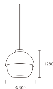
OK 30071 28000 Φ300*H280mm 線長: 1500mm E27*1 另計 鋼材 玻璃
