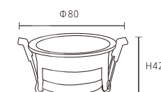
JBR-31081B/W 尺寸 \Phi 80 \times H42 mm 開孔尺寸 \Phi 75
