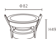
JBR-31072 尺寸 \Phi 82 \times H49 mm 開孔尺寸 \Phi 75 可適用MR16
