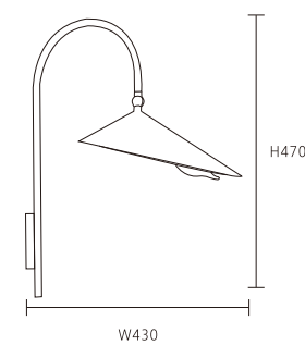
OK 31551/31552 35000 W430*H470mm 線長:1000mm E14*1 另計 鋼材 電源線附按鈕開關
