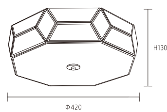
OK 31672 48000 Φ420*H130mm E27*3 另計 全銅 玻璃
