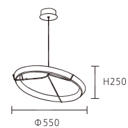
OK 30492 92000 \Phi 550 \times H250 mm 線長:1500mm 內附 LED 32W 3000K 金屬 壓克力
