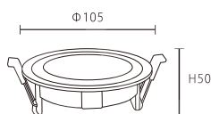
JBR-31078 尺寸 \Phi 105 \times H50 mm 開孔尺寸 \Phi 95 可適用MR16
