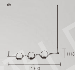
OK 30521 86000 L1300*H180mm 線長: 1500mm E14*3 另計 全銅 玻璃
