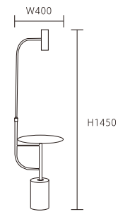
OK 31771 106000 W400*H1450mm 線長:1000mm 內含 LED 5W 三段光色 鋼材 大理石
