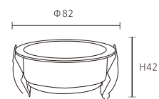
JBR-31091B/W 尺寸 \Phi 85 \times H 42 \text{mm} 開孔尺寸 \Phi 80 可適用MR16 前置式光源
