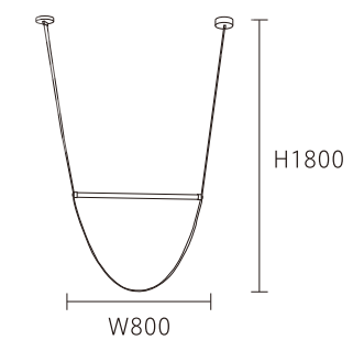
OK 30421 80000 W800*H1800mm 內附 LED 14W 3000K 壓克力 灰色皮革 單邊可裁切
