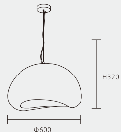
OK 30032 87000 Φ600*H320mm 線長: 1500mm E27*1 另計 樹脂
