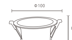
JBR-31083B/W 尺寸 \Phi 100 \times H42 mm 開孔尺寸 \Phi 95
