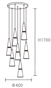
OK 30891 120000 Φ400*H1700mm 線長:1500mm 內附 LED 5W*7 3000K 鋼材 清光玻璃
