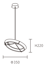
OK 30491 75000 \Phi 350 \times H220 mm 線長:1500mm 內附 LED 20W 3000K 金屬 壓克力
