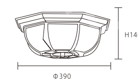
OK 31682 50000 Φ390*H140mm E27*3 另計 全銅 玻璃
