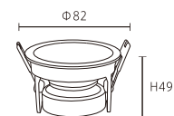
JBR-31073 尺寸 \Phi 82 \times H49 mm 開孔尺寸 \Phi 75 可適用MR16
