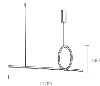
OK 30642 85000 L1200*D400mm 線長: 1500mm 內附 LED 30W 4000K 不銹鋼 壓克力
