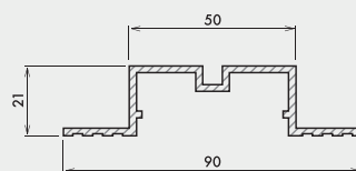
PROFILO MONTANTE - ART. P70289
