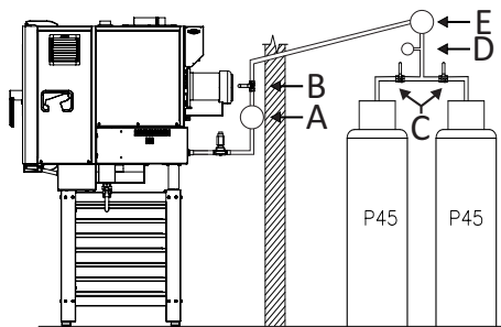
Tubería de etapa superior a 10m
