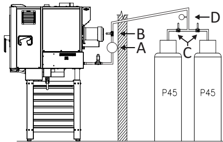
Tubería de etapa inferior a 10m
