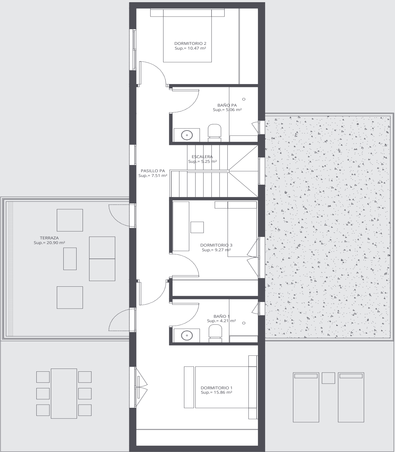
PLANTA ALTA
