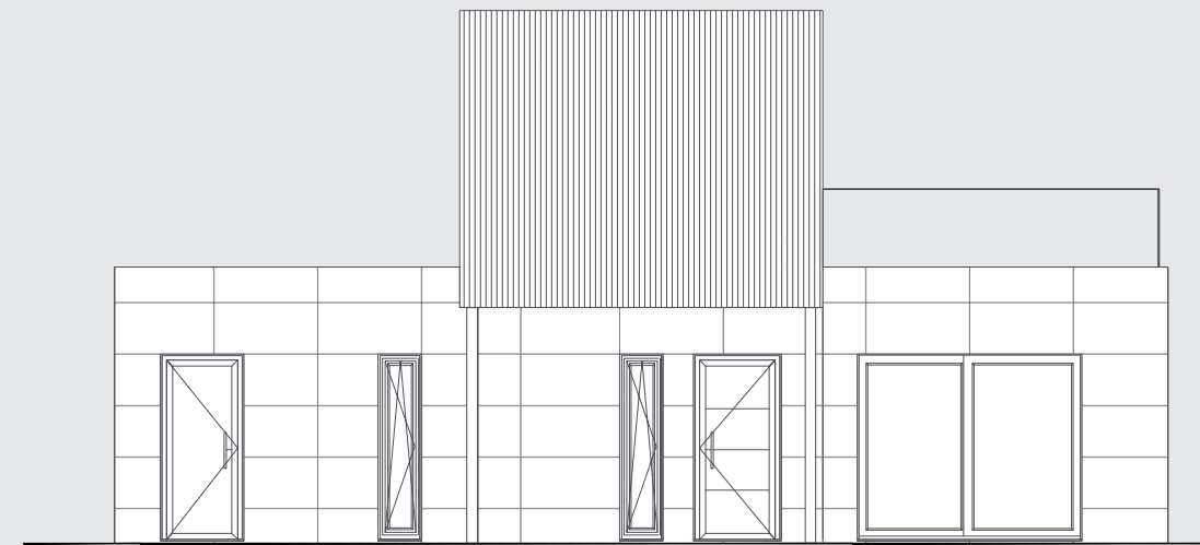
ALZADO C
