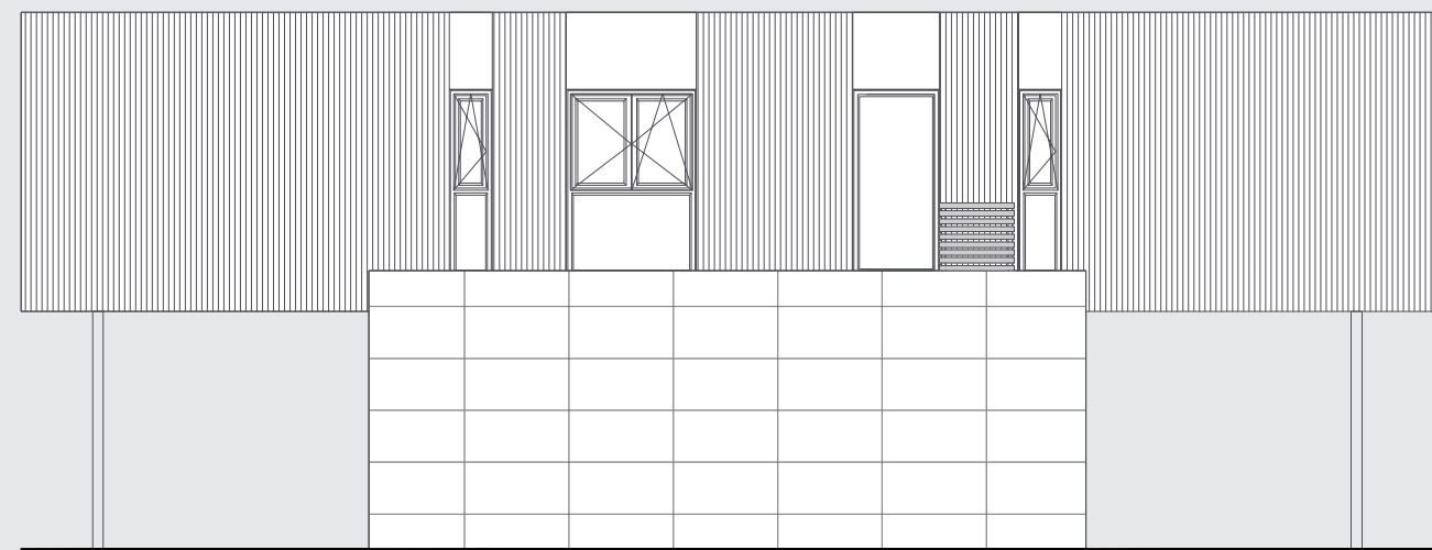
ALZADO B
