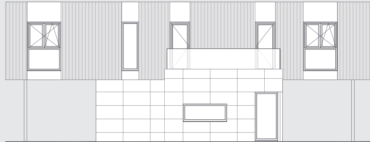
ALZADO A
