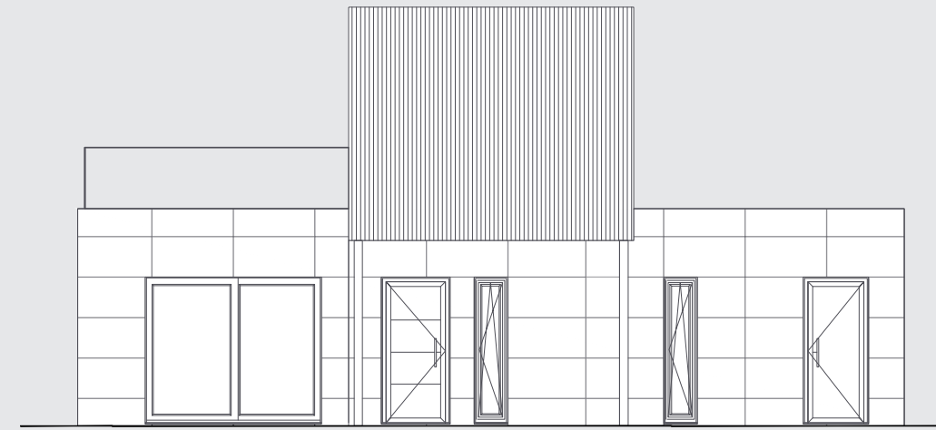
ALZADO C
