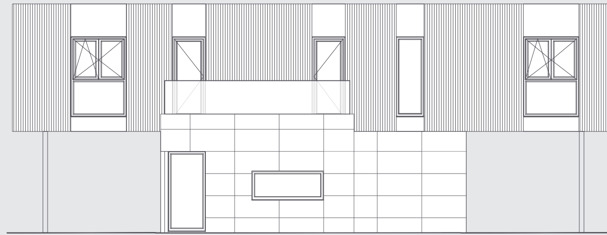
ALZADO A
