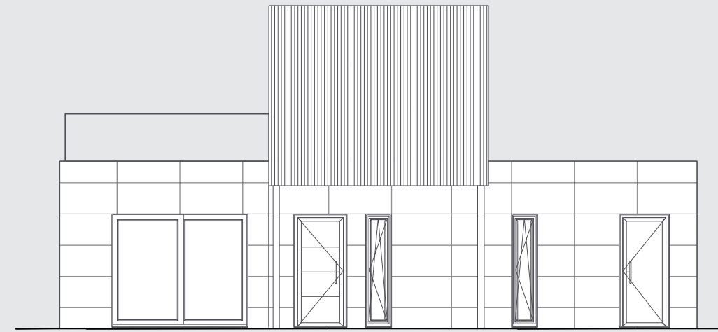
ALZADO C
